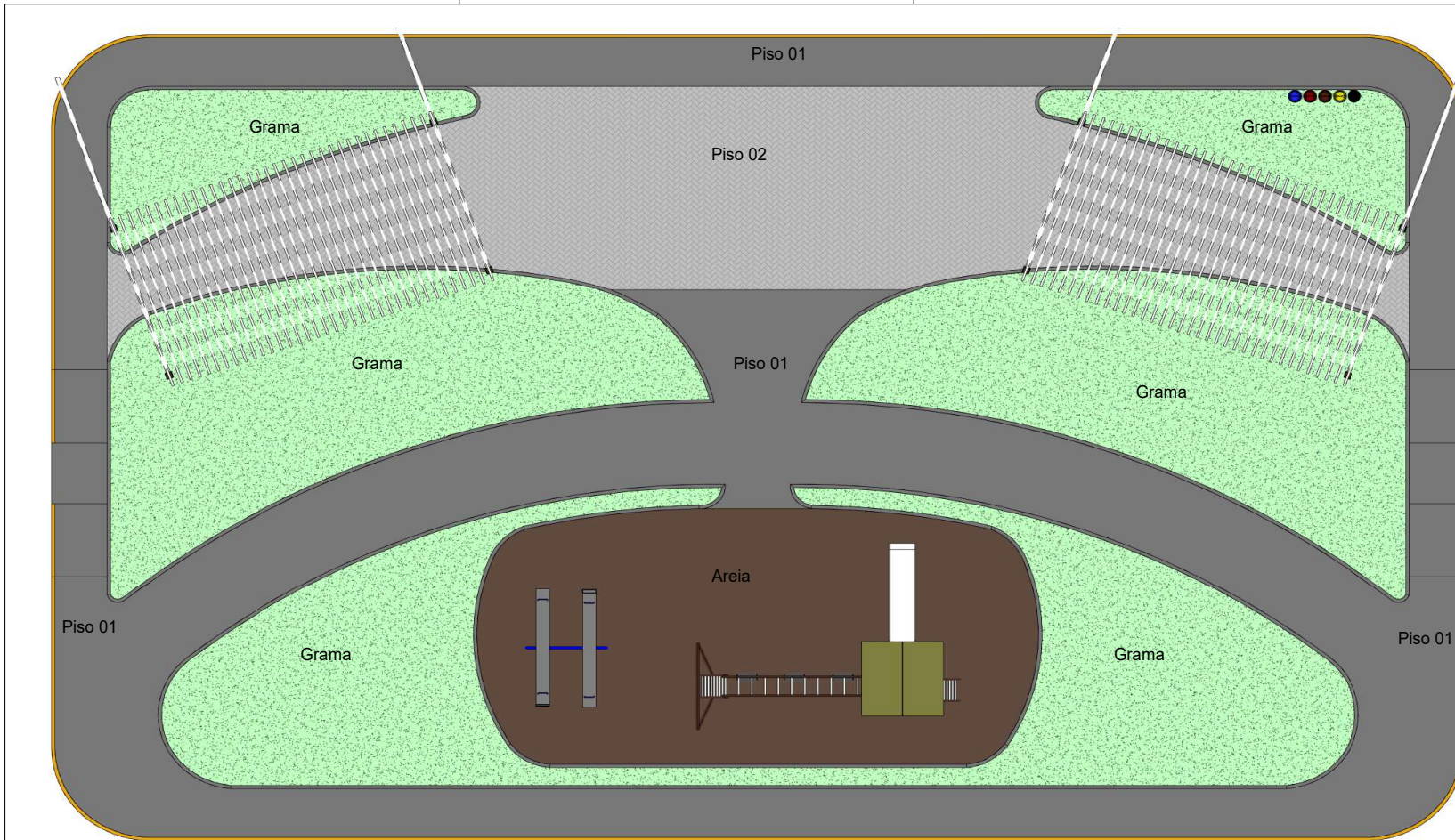
1 PLANTA DE LAYOUT 1 : 100
