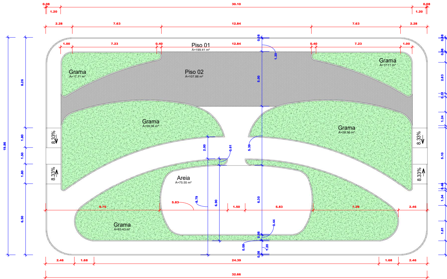
1 PLANTA DE COTA 1 : 125
